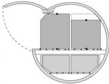
Porão de carga carregado lateralmente
