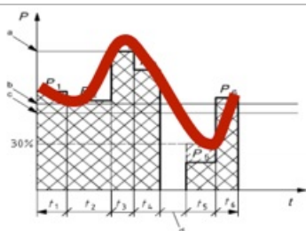
Carga Variável
